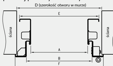
przekrój poziomy ościeżnicy w murze
