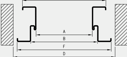
przekrój poprzeczny
