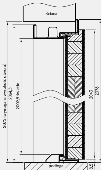
przekrój pionowy drzwi Forca
