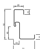
Rysunek techniczny
