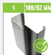
Ościeżnica „9” lub „11” laminowana z uszczelką
