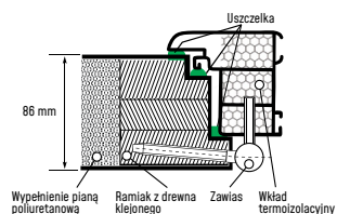
PROFIL SKRZYDŁA TERMO PRESTIGE LUX
