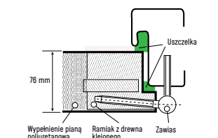
PROFIL SKRZYDŁA OPTIMUM
