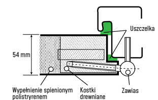
PROFIL SKRZYDŁA NORMAL
