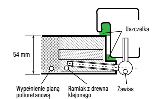
PROFIL SKRZYDŁA PREMIUM
